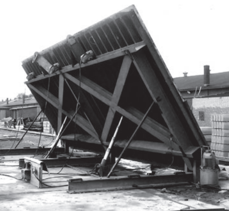
Construcción de mesa basculante con diagonales cruzadas
