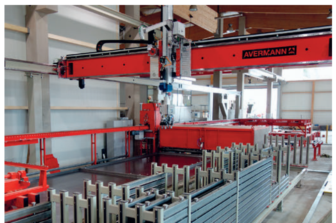
Robot de encofrado
